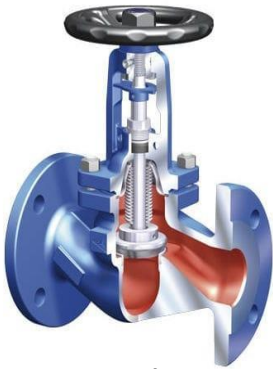
Robinetts à soufflet Manuels ou Motorisables FABA PLUS 046 & SUPRA I
