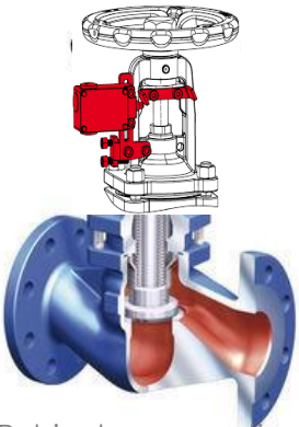
Robinetts avec options fins de course, volant à chaîne, clapets PTFE et d'équilibrage
