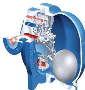
Pompe à condensat CONA P
