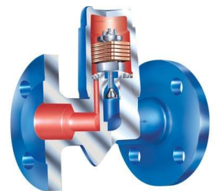
Purgeurs toutes technologies CONA - M / B / S
